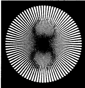
Abb. 8b Aufnahme eines Siemenssterns durch ein um 0,5 dpt defokussiertes Fernglas mit Dachprisma bei Phasenverschiebung um eine halbe Wellenlänge zwischen den Pupillenhälften
