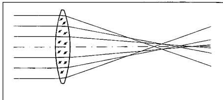
Abb. 1 Beispiel für Abbildungsfehler: Öffnungsfehler an der Einzellinse
