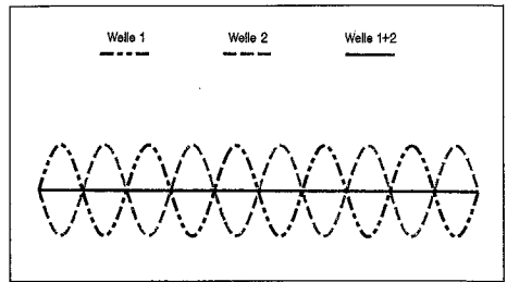
Abb. 3b Lichtauslöschung durch Interferenz
