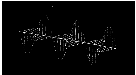
Abb. 5a Parallel und senkrecht schwingende Lichtwelle vor der Totalreflexion
