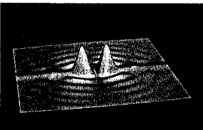
Abb. 6a Lichtverteilung im Bild eines leuchtenden Punktes bei Phasenverschiebung um eine halbe Wellenlänge zwischen den Pupillenhälften
