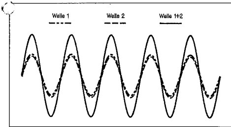
Abb. 3a Lichtverstärkung durch Interferenz
