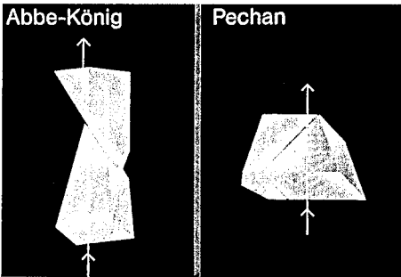
Abb. 4a Dachprisma nach Abbe-König Abb. 4b Dachprisma nach Pechan
